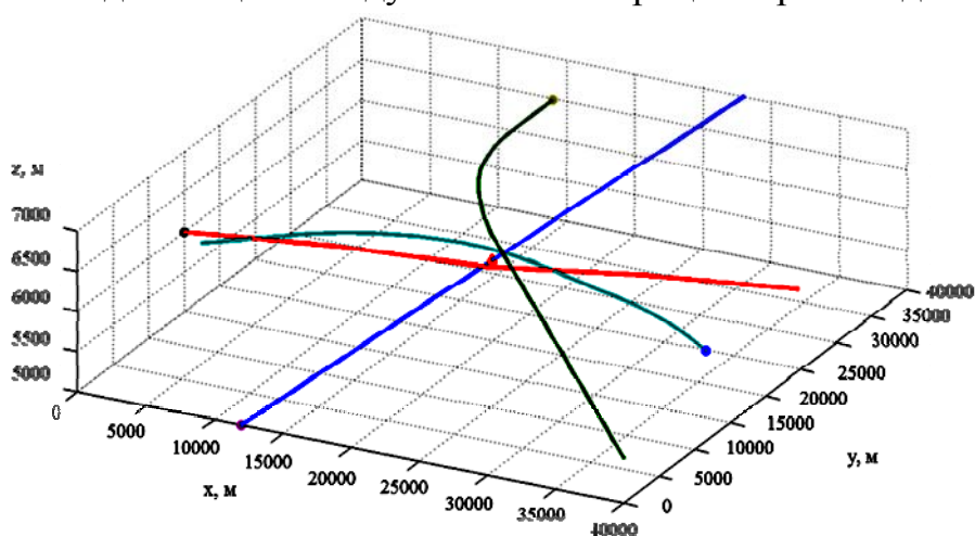
Рис. 1. Результаты моделирования угрозы столкновения четырех самолетов
