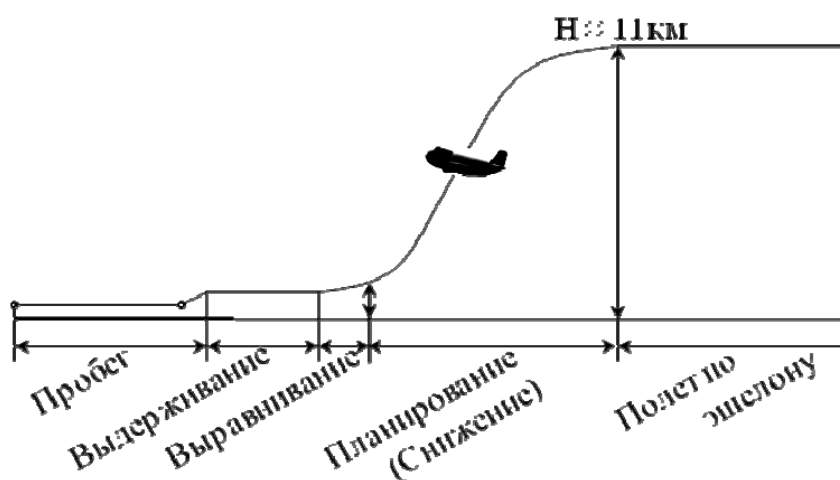
Рис. 2. Схема этапов посадки самолета по криволинейным предельным траекториям
